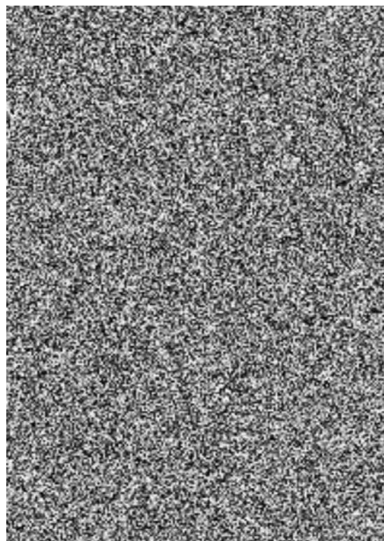
Figura 8. Imagen PGM recuperada para una diferencia \Delta\varepsilon_{11} = 10^{-16} .
