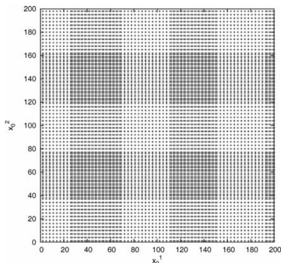
Figura 3. Conjunto de semillas que producen en 25 iteraciones el par (b_{25}^1, b_{25}^2) = (1,1) para \varepsilon = 0 .
