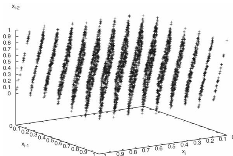
Figura 1. Mapa de retorno tridimensional para RANDU ( 2^{31} , 65539, 0, x_0 ).
