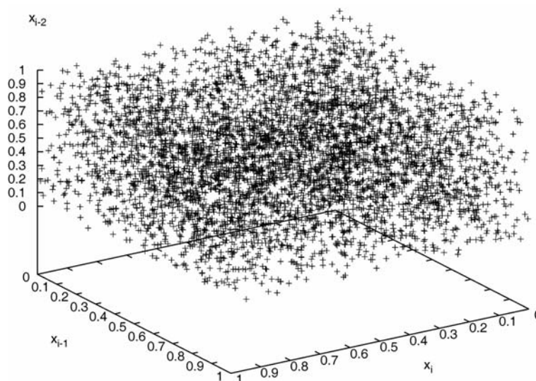
Figura 2. Mapa de retorno tridimensional para el caso de 2 GCLs RANDU ( 2^{31} , 65539, 0, x_0 ) idénticos acoplados.
