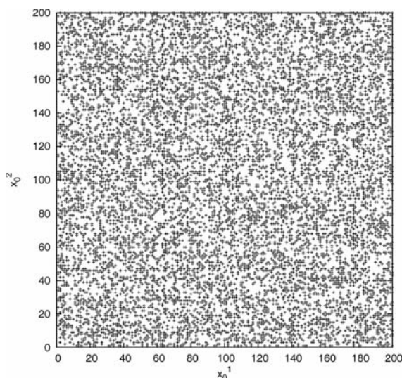
Figura 4. Conjunto de semillas que producen en 25 iteraciones el par (b_{25}^1, b_{25}^2) = (1,1) para \varepsilon = 10^{-5} .
