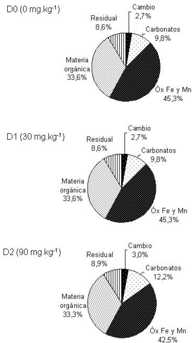
Figura 2. Distribución del níquel en las diferentes fracciones químicas.
